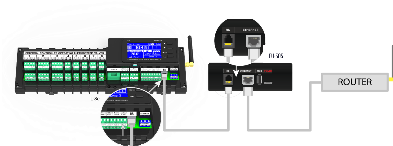
Kapcsolási rajz az EU-505 internetes modulhoz.
