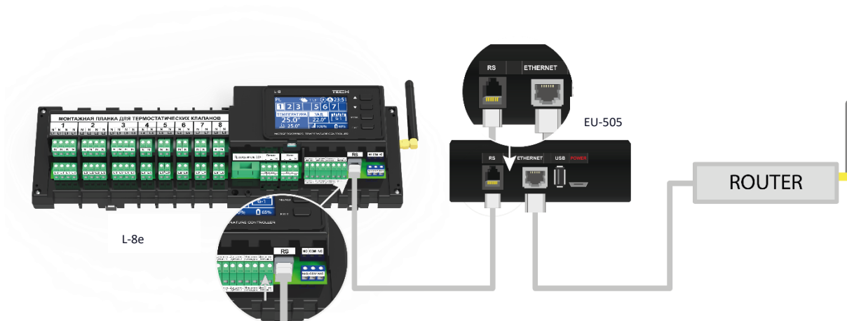
Схема подключения Интернет-модуля EU-505.
