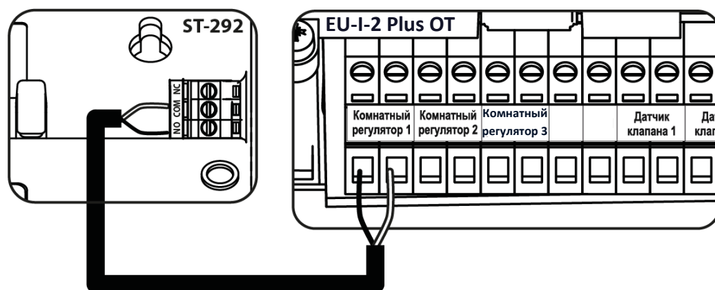
Примерное подключение двухрежимного регулятора
