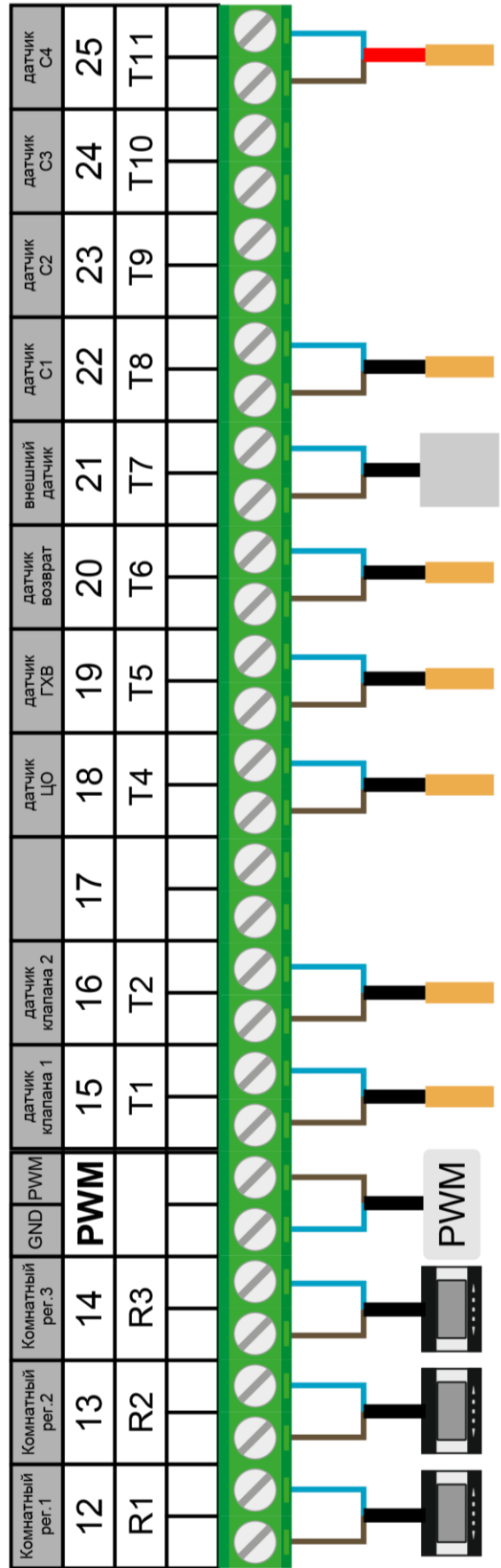
Разъемы, символы и пример использования
