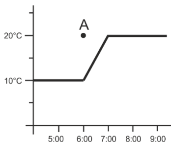
Raumtemperatur – bei ausgeschalteter Funktion „OPTIMUM START“
