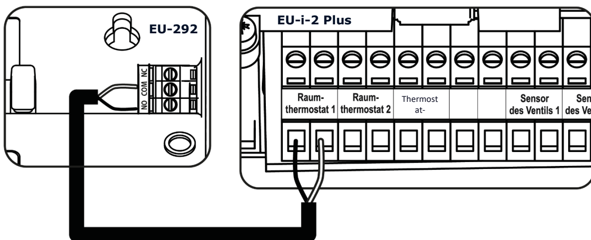
Beispielhaftes Anschließen eines Zweipunktreglers
