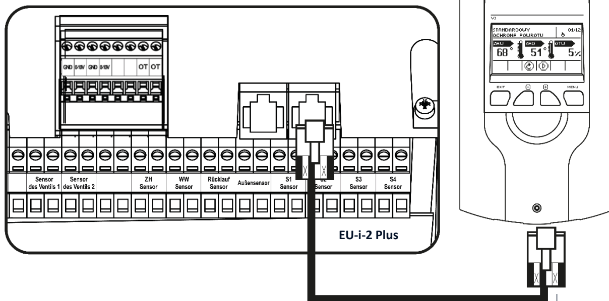
Beispielhaftes Anschließen des Zusatzventils mit dem Hauptsteuergerät EU-i-2 Plus
