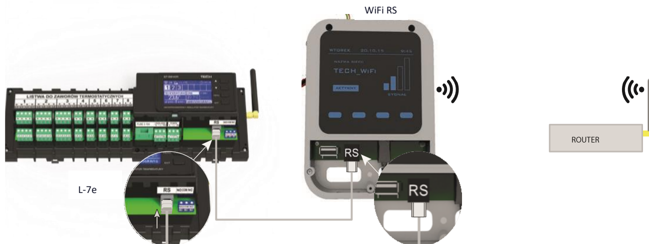
Schéma připojení internetového modulu WiFi RS.
