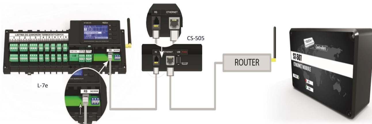
Schéma připojení internetového modulu CS-505.
