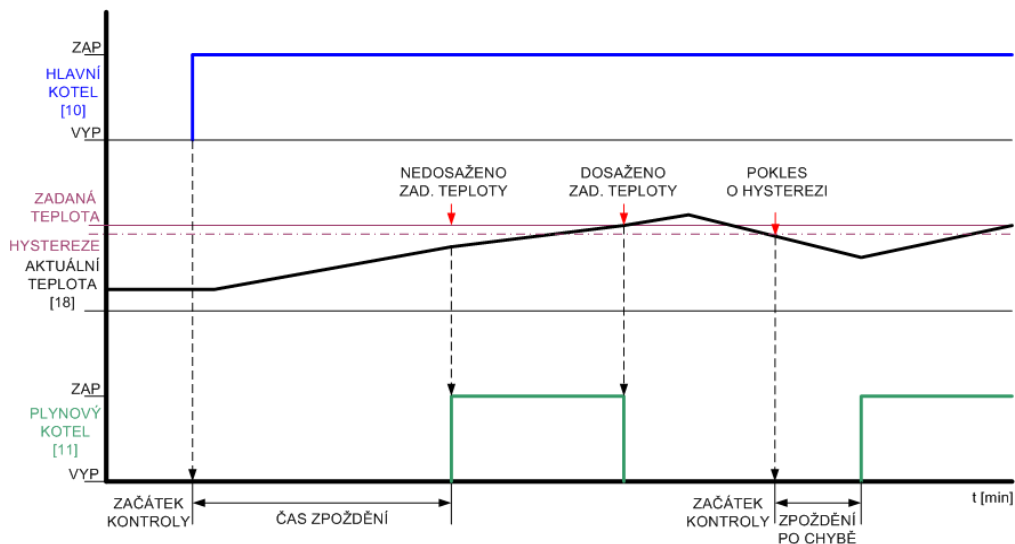
Grafické znázornění algoritmu Kontrola provozu .
