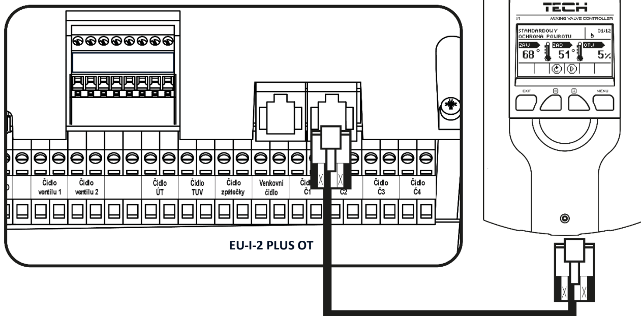
Příklad propojení modulu CS-i-1 s hlavním regulátorem EU-i-2 Plus OT
