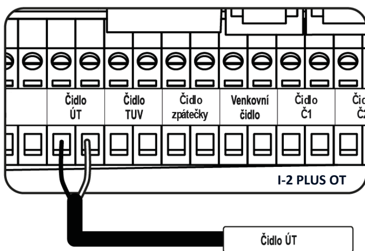
Připojení čidla ÚT
