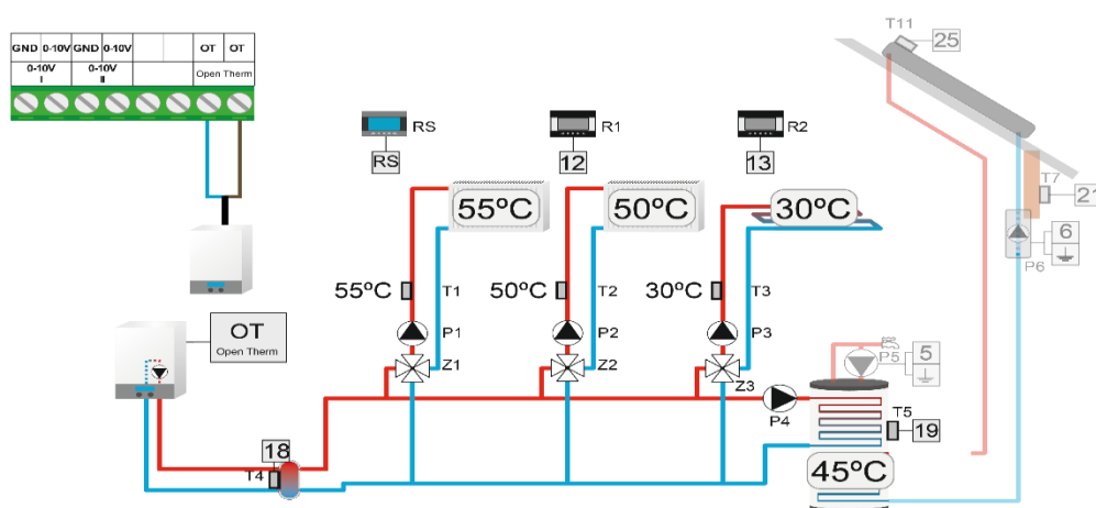
Příklad zapojení instalace Open Therm.
